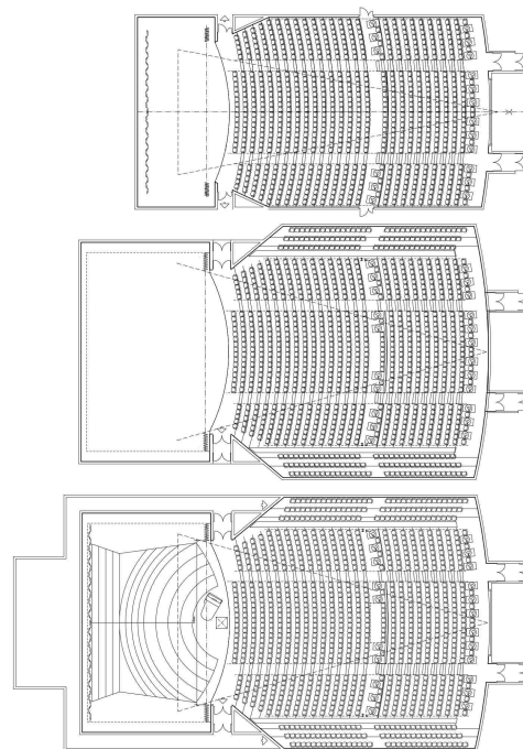
Gabarit de faisabilité de la salle 1000 en phase programme
