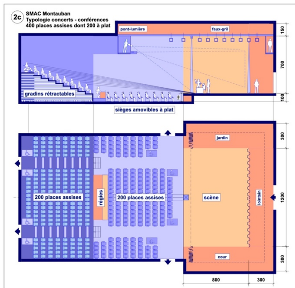
Schémas des diverses typologies salle/scène/régies
