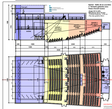
Épures de gabarit de l'auditorium
